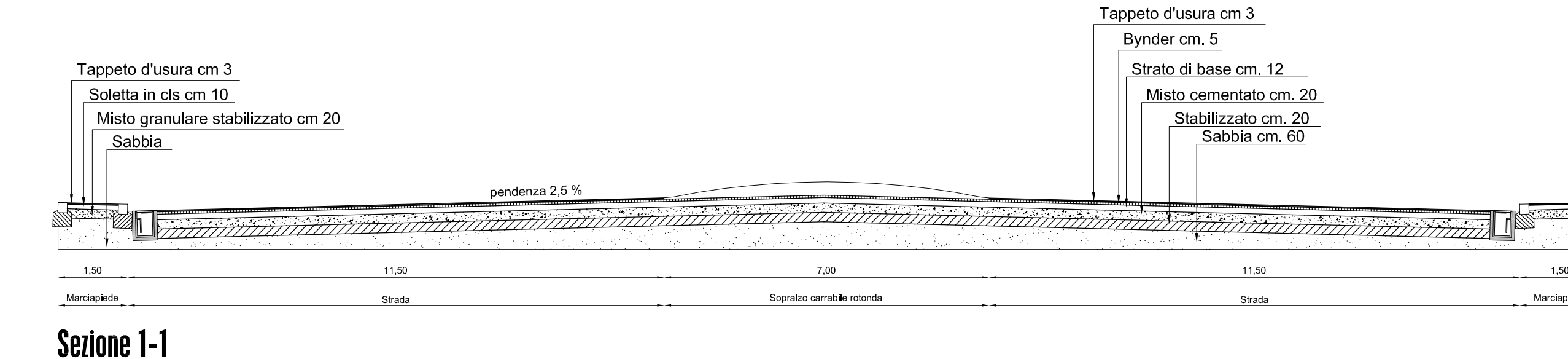
Sezione 1-1
