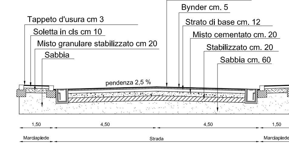
Sezione 5-5
