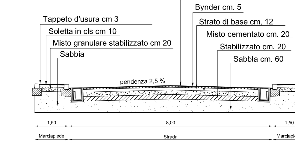
Sezione 7-7
