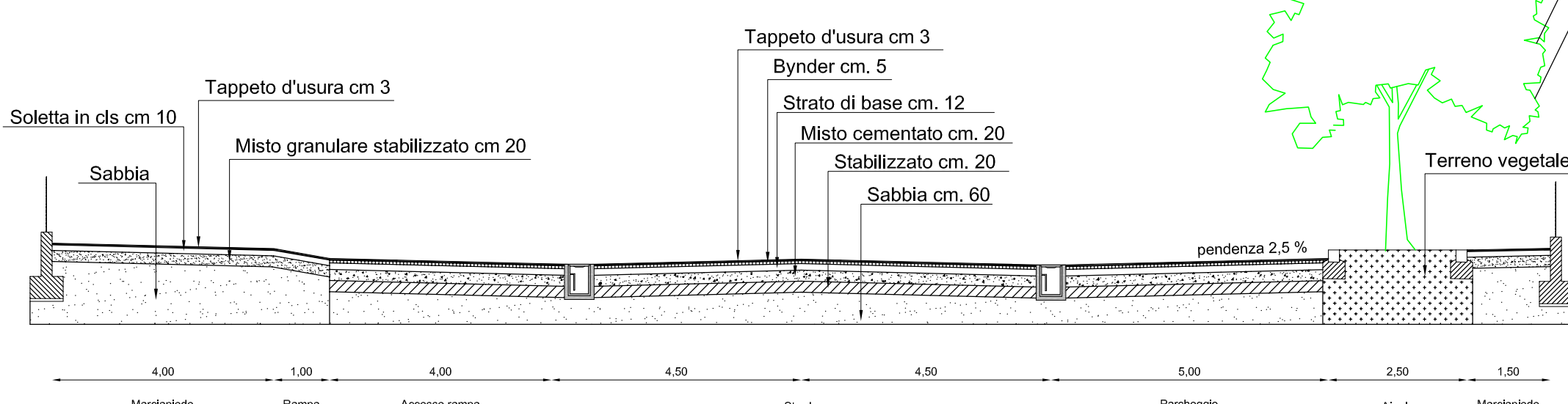
Sezione 2-2
