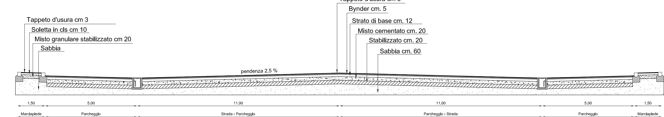
Sezione 4-4
