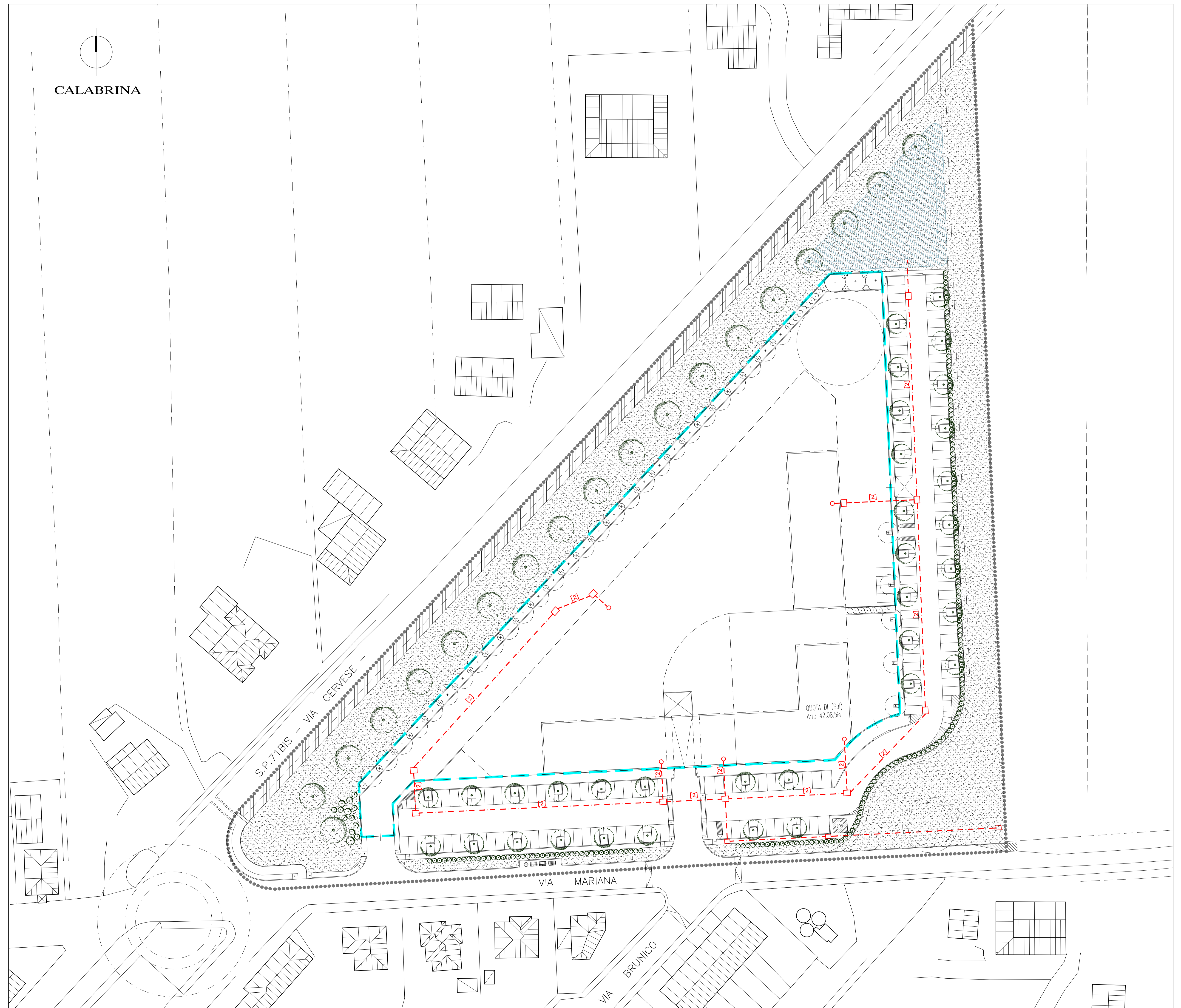
PLANIMETRIA 1:500
