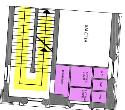
PIANTA PIANO AMMEZZATO
