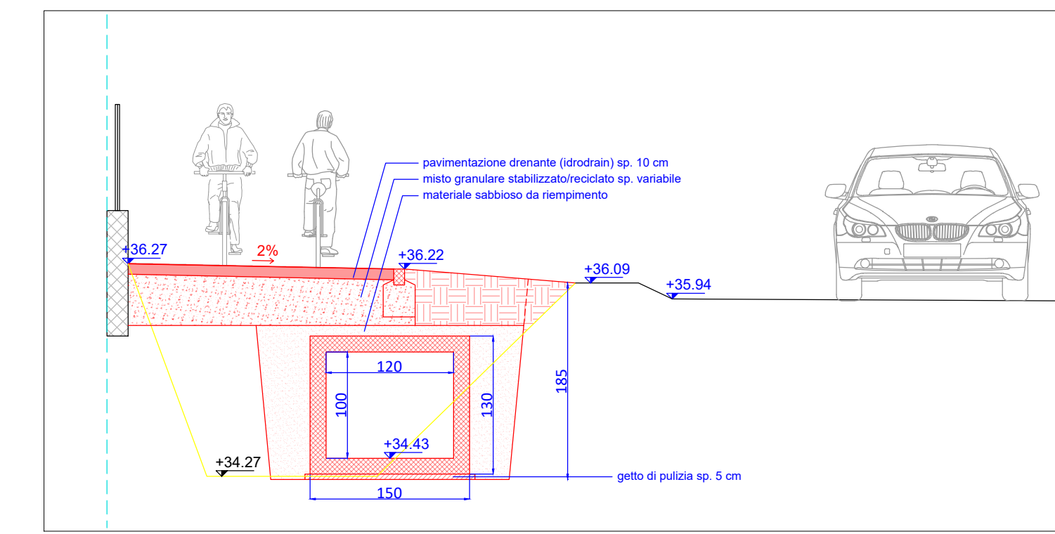
sez E-E_rapp. 1:50
